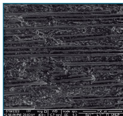
Figura 2. Perno de fibra translúcido. Microestructura.
